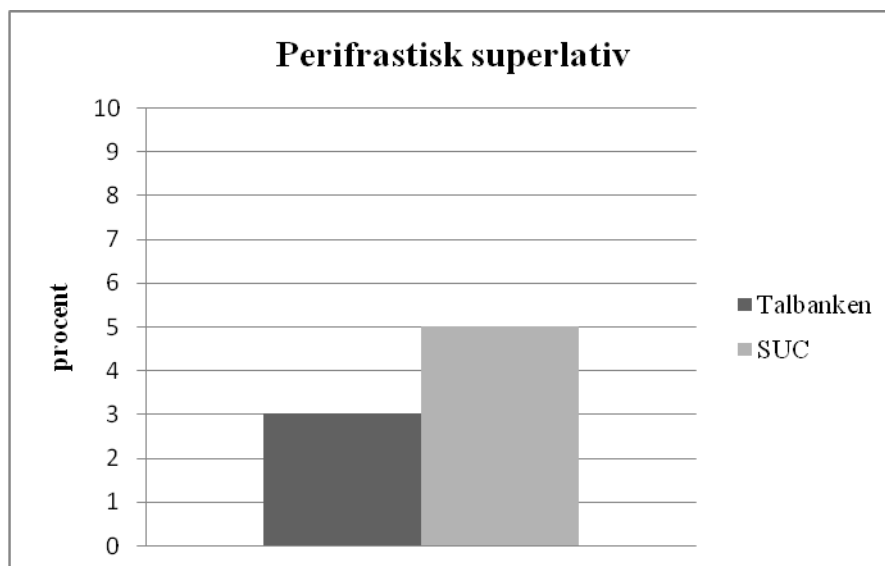
Figur 2. Andelen perifrastiska superlativer i Talbanken och SUC.
