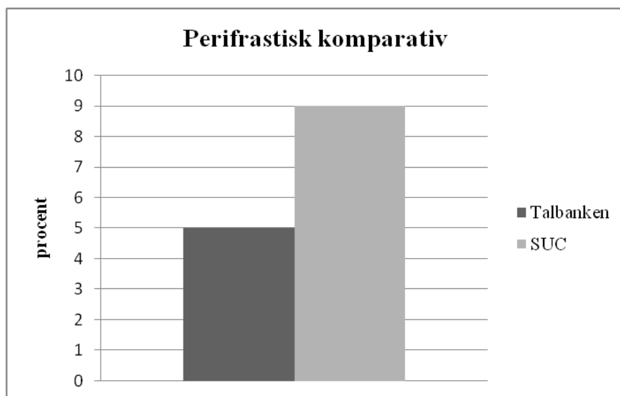
Figur 1. Andelen perifrastiska komparativer i Talbanken och i SUC.
